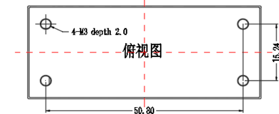
整机型 60.1*25.4*12.7mm
