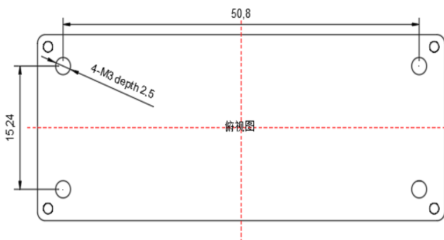
标准型 58.1mm*23.0mm*9.8mm
