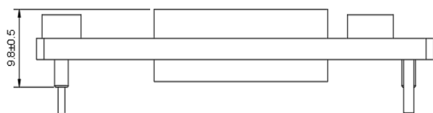
标准型 58.1mm*23.0mm*9.8mm
