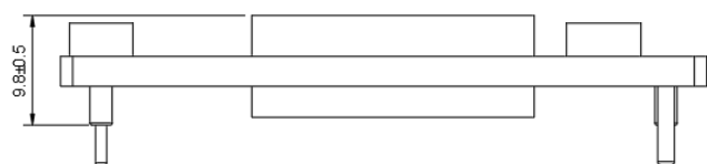
标准型 58.1mm*23.0mm*9.8mm
