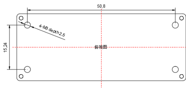
标准型 58.1mm*23.0mm*9.8mm
