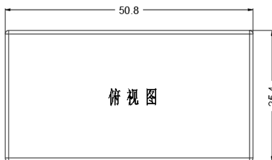
标准型 50.8*25.4*12.7mm
