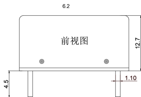
标准型 25.4*25.4*12.7
