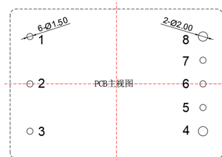
推荐PCB开槽尺寸
