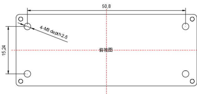
标准型 58.1mm*23.0mm*9.8mm
