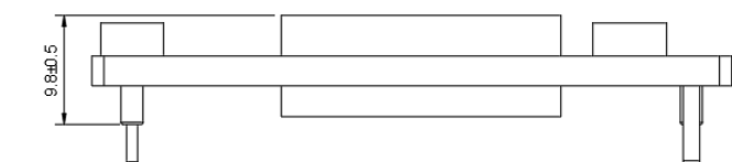
标准型 58.1mm*23.0mm*9.8mm
