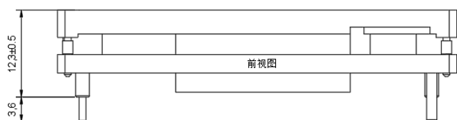
标准型+散热铝板 58.1mm*23.0mm*12.3mm
