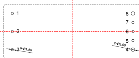
推荐PCB开槽尺寸
