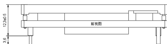
标准型+散热铝板 58.1mm*23.0mm*12.3mm
