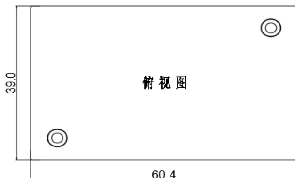
标准型 60.4*39.0*12.7mm
