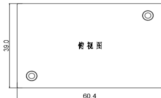
标准型 60.4*39.0*12.7mm
