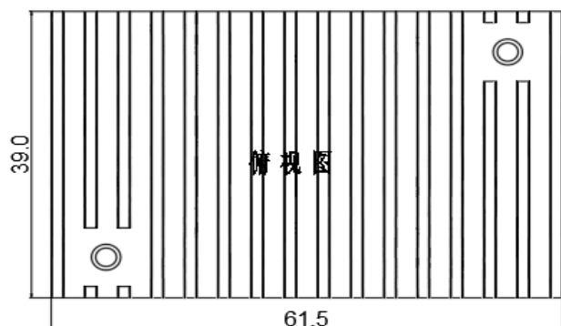
标准型+散热器 61.5*39.0*27.7mm
