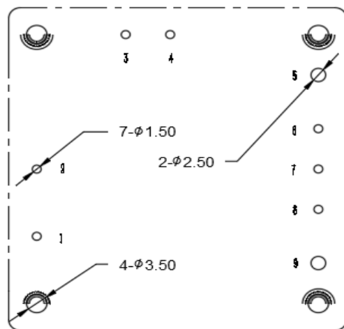
推荐PCB开槽尺寸
