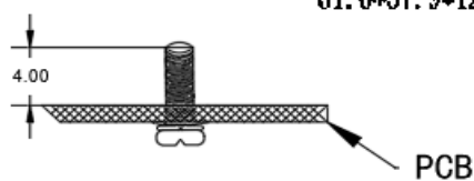
标准型 61.0*57.9*12.7mm
