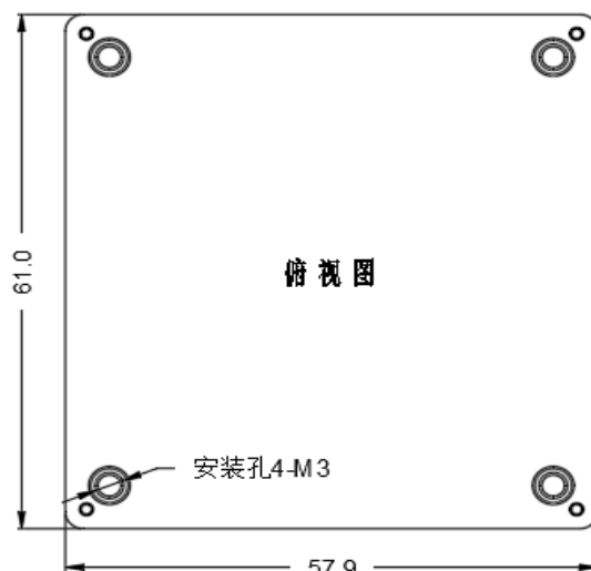
标准型 61.0*57.9*12.7mm
