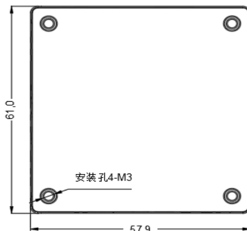
标准型 61.0*57.9*12.7mm
