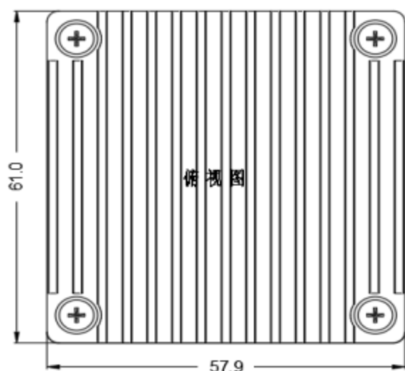
标准型+散热器 61*57.9*27.7mm
