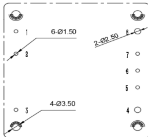
推荐PCB开槽尺寸
