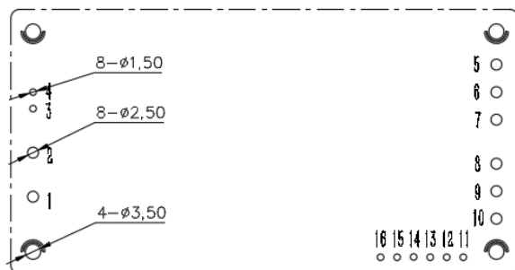
推荐PCB开槽尺寸
