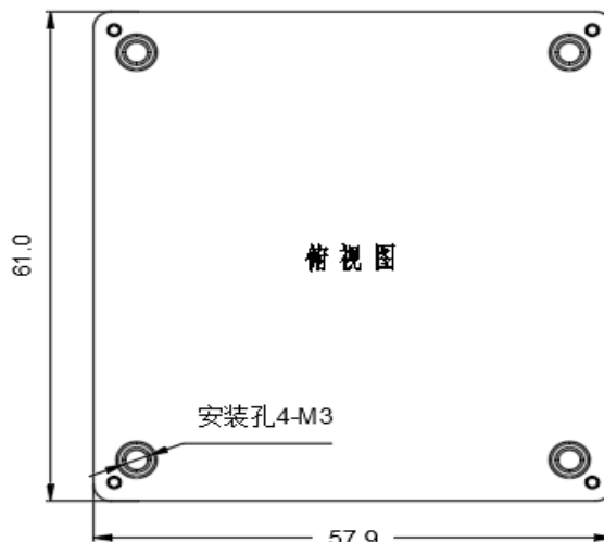
标准型 61.0*57.9*12.7mm
