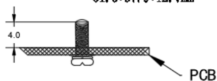
标准型 61.0*57.9*12.7mm
