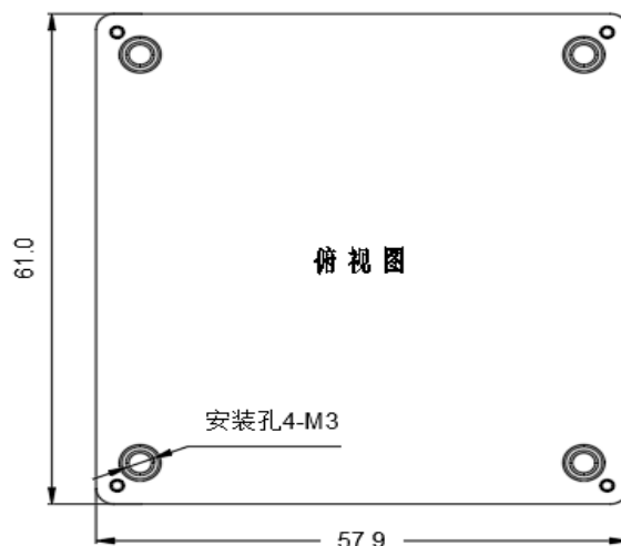
标准型 61.0*57.9*12.7mm
