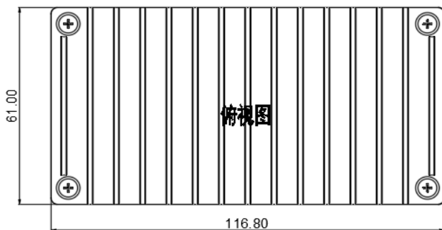
标准型+散热器 116.8*61.0*32.7mm
