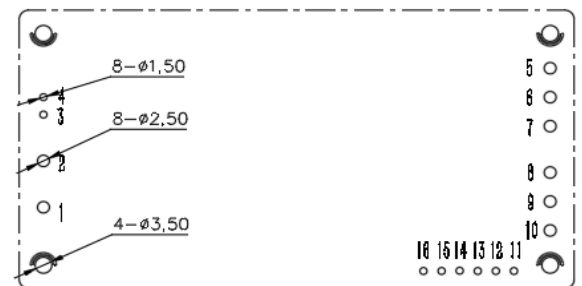
推荐PCB开槽尺寸
