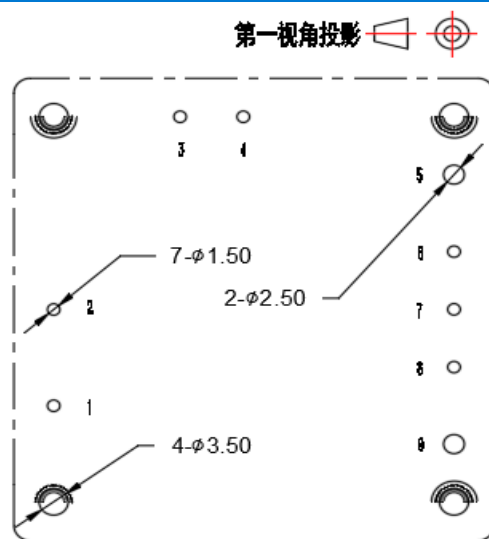
推荐PCB开槽尺寸
