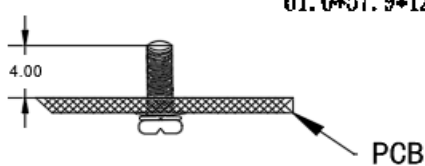
标准型 61.0*57.9*12.7mm
