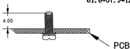
标准型 61.0*57.9*12.7mm
