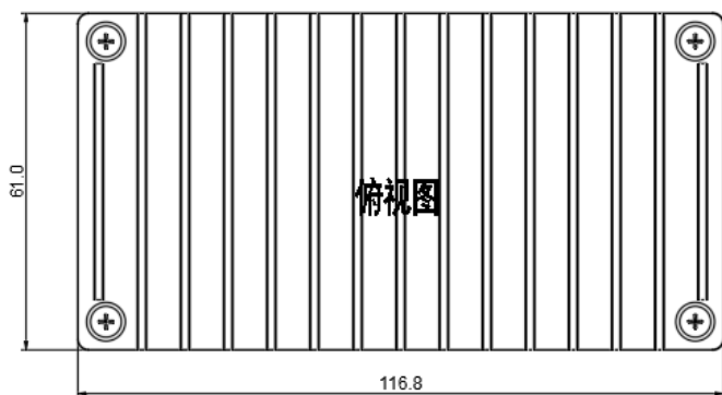
标准型+散热器 116.8*61.0*32.7mm
